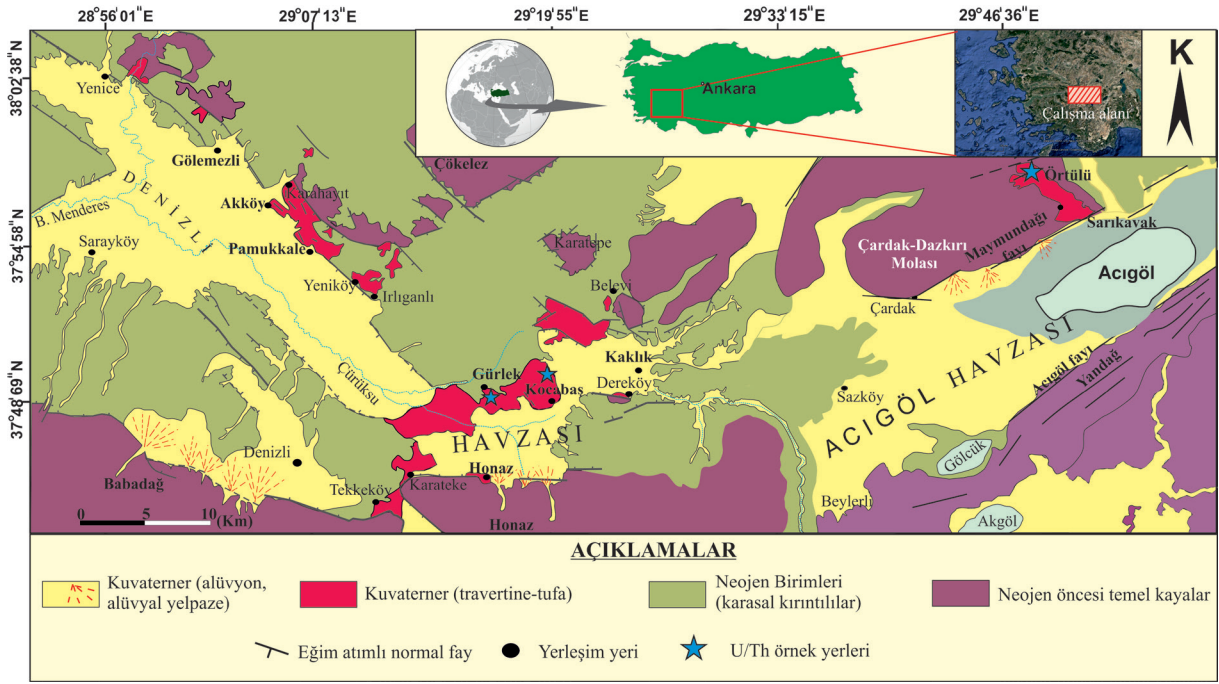
Şekil 1. Denizli ve Acıgöl Havzalarının basitleştirilmiş jeolojisi haritası ve karasal karbonat çökellerinin (travertine-tufa) dağılımı (Sun, 1990).
